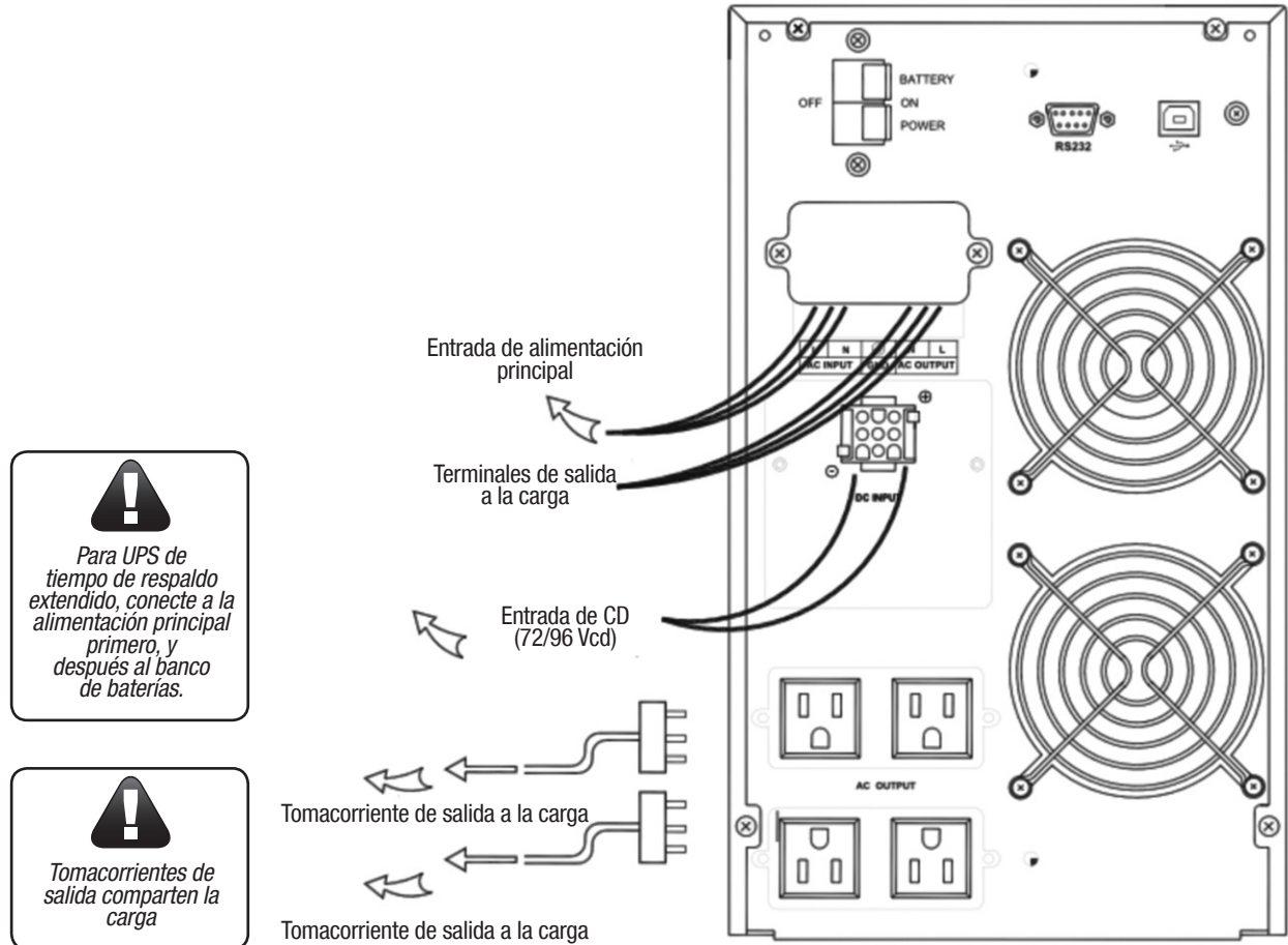
Fig. 4-3 Esquemático de conexiones del UPS-IND 1118 y UPS-IND 1122
