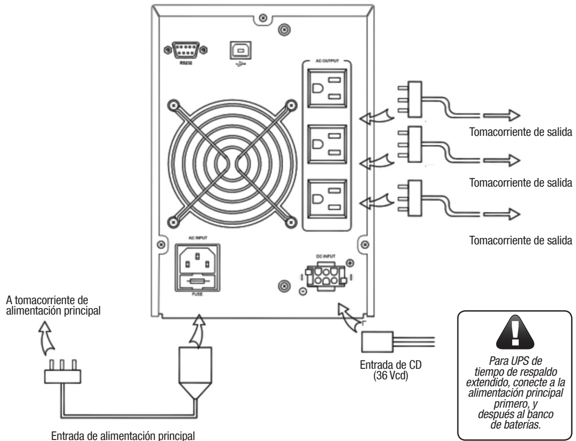
Fig. 4-2 Esquemático de conexiones del UPS-IND 1110
