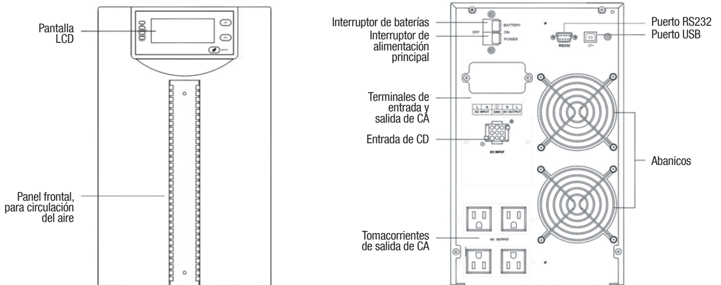
Fig. 2-3 Estructura del panel frontal y posterior del UPS-IND 1118 y UPS-IND 1122
