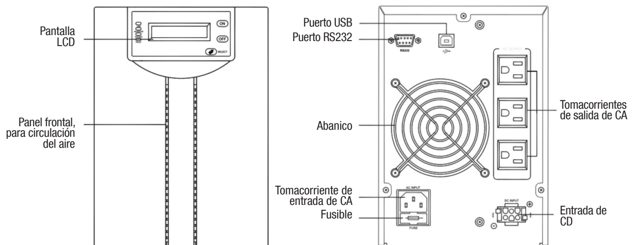
Fig. 2-2 Estructura del panel frontal y posterior del UPS-IND 1110
